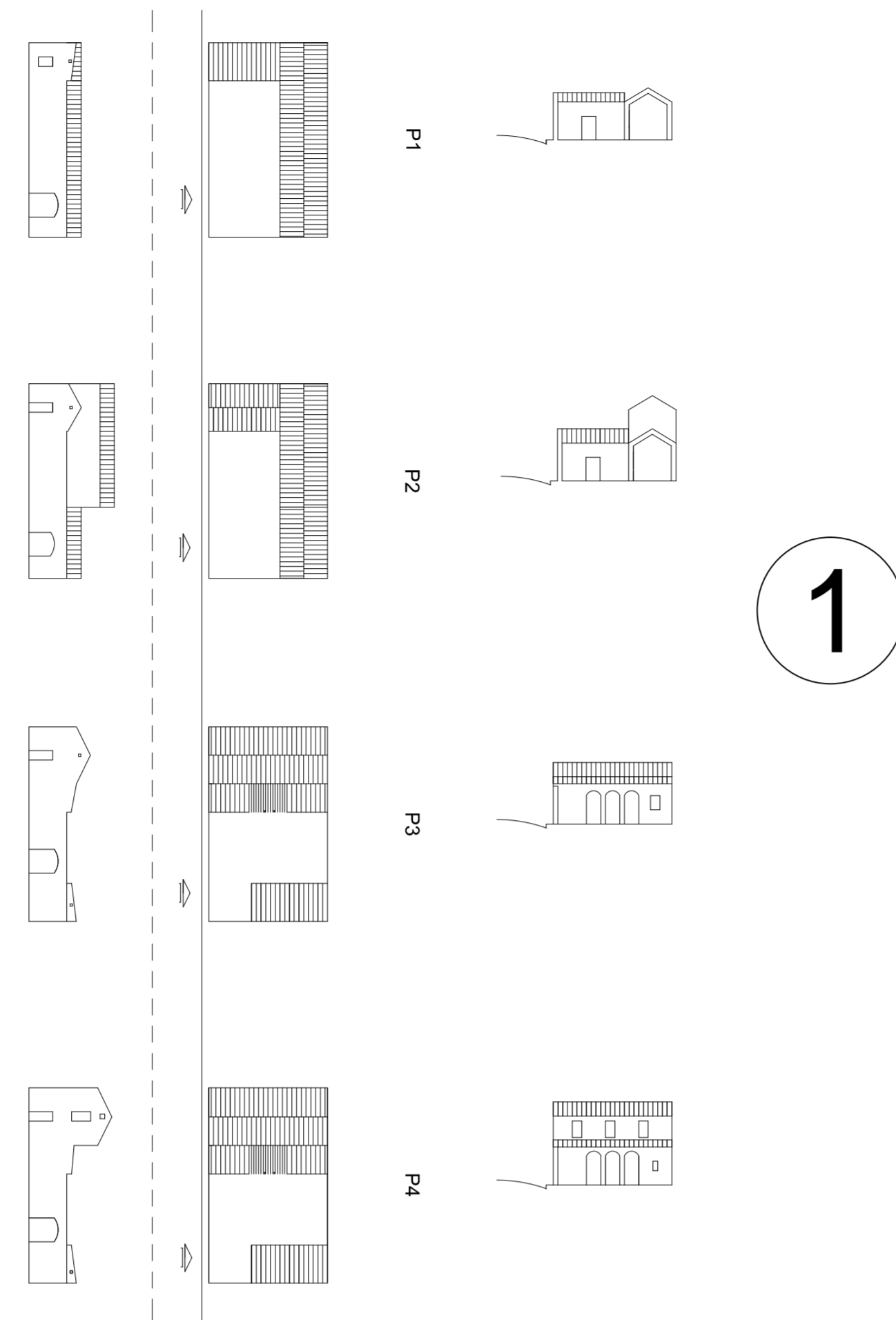
CORTI PICCOLE IN LUNGHEZZA E ACCESSO DA SUD E LATERALE
