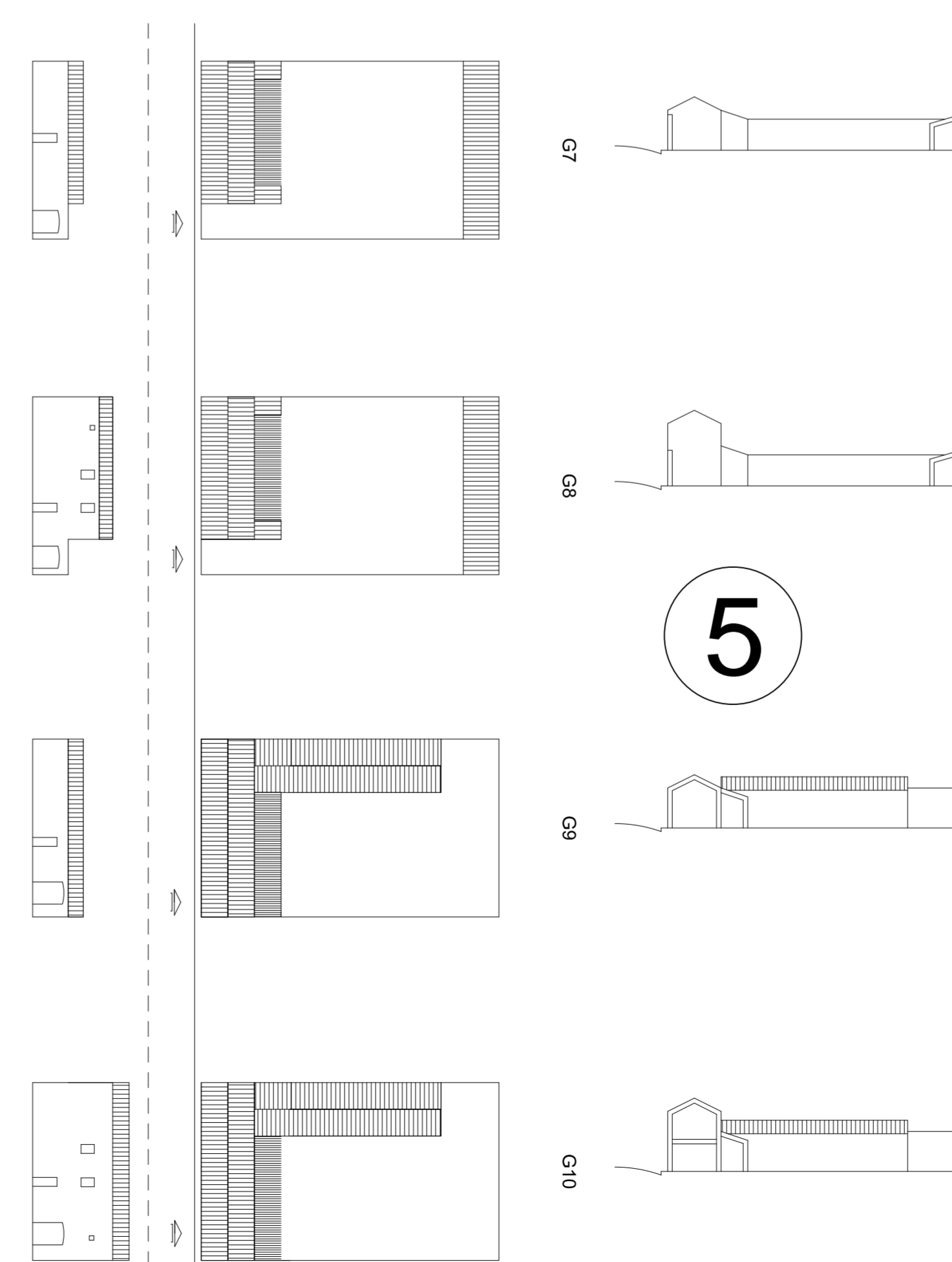
CORTI GRANDI CON ACCESSO DA NORD E LATERALE
