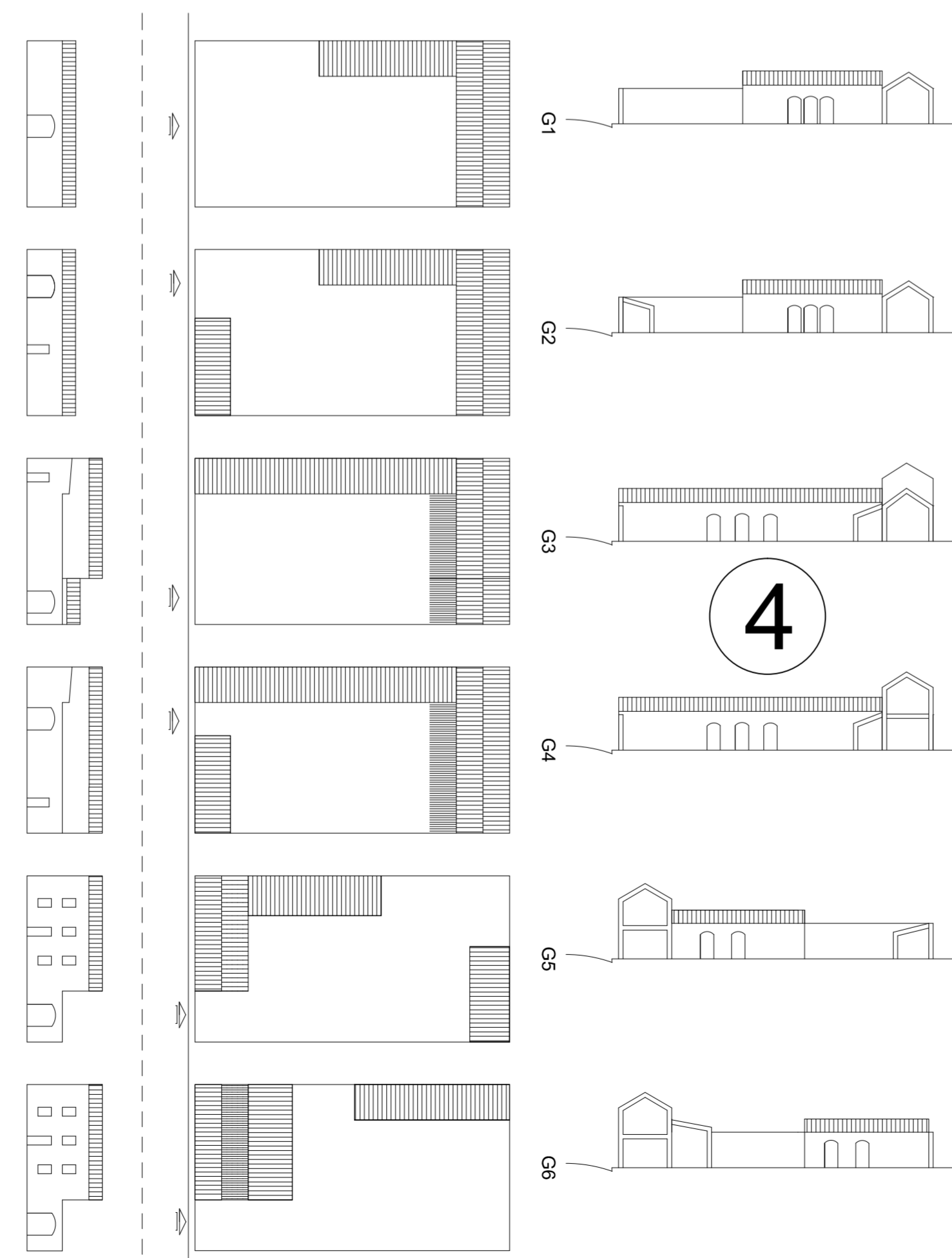
CORTI GRANDI CON ACCESSO DA SUD E LATERALE
